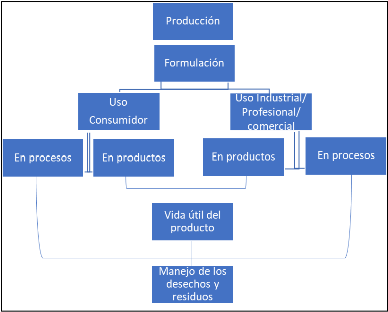
FIGURA 2. ETAPAS DEL CICLO DE VIDA QUE PODRÍAN INCLUIRSE EN UNA EVALUACIÓN DE RIESGOS COMPLETA. FUENTE: ICCA (2011) CON MODIFICACIONES
